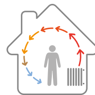
Convectie
